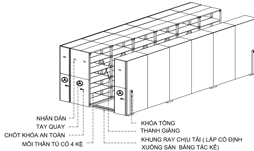
HÌNH CHIẾU TRỰC ĐO
