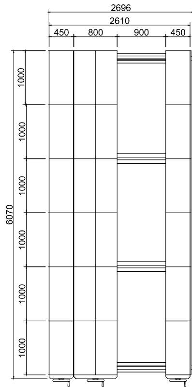
HÌNH CHIẾU BẰNG
